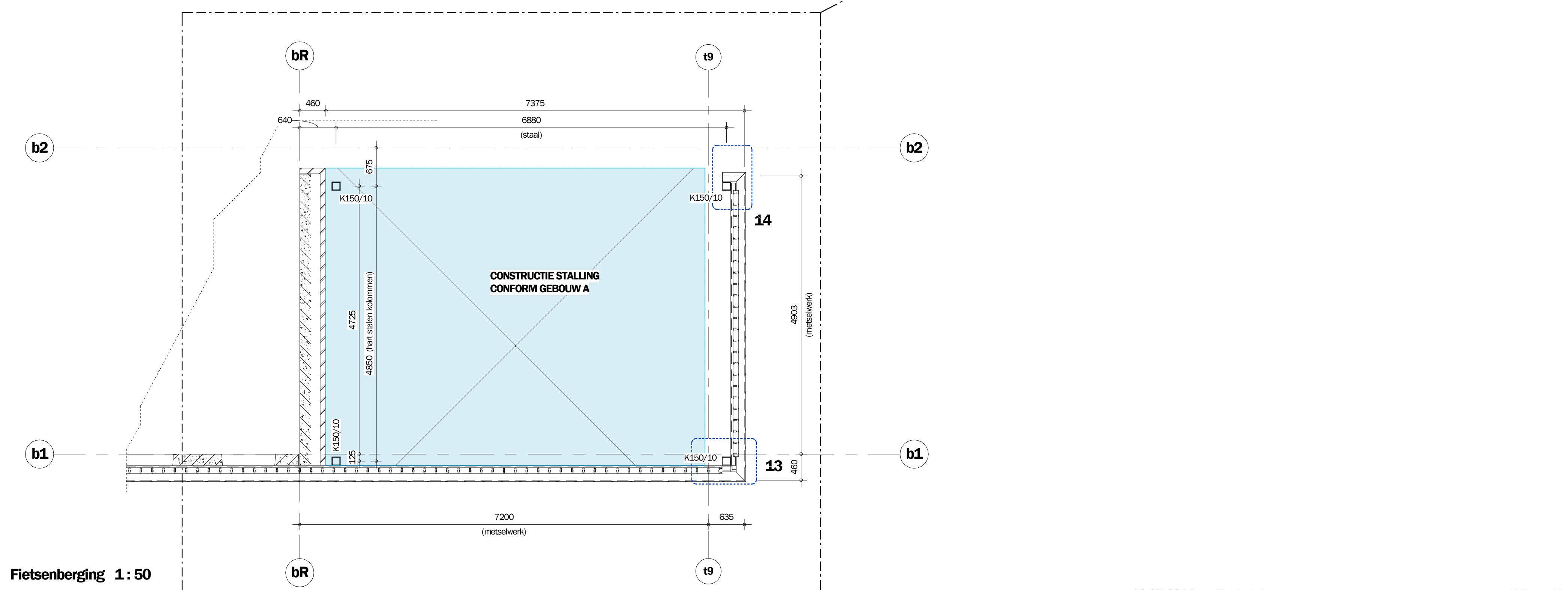
Fietsenberg 1:50
